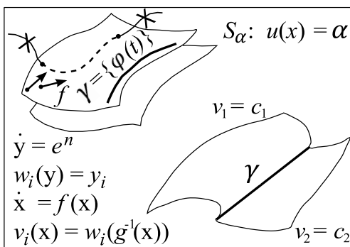
Рис. 3.2. Первые интегралы
