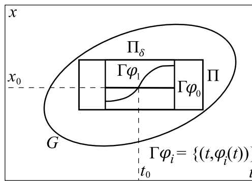
Рис. 2.2. Приближения \varphi
