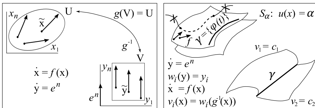
Рис. 3.1. Выпрямление поля f
