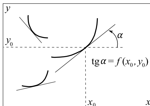
Рис. 1.2. Поле направлений
