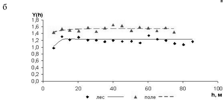
Рис. 2. Вариограммы для почвенных свойств (точки – экспериментальные данные, линии – модель): а – pH, б – содержание органического углерода
