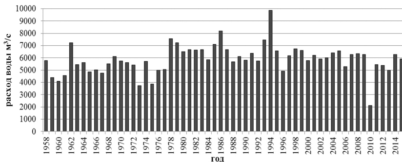
Рис. 5. Изменения величины осредненных расходов за август
