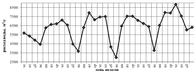
Рис. 2. Характерное колебание расходов воды на ГЭС в зависимости от дня недели (июль 1999 г.)
