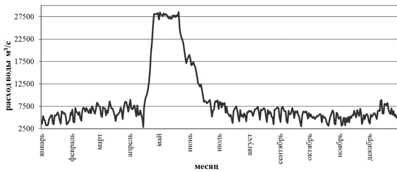
Рис. 1. Сезонное и недельное регулирование водного стока Жигулевской ГЭС в 2002 г. (гидрологические данные предоставлены филиалом «РусГидро» – Жигулевская ГЭС)
