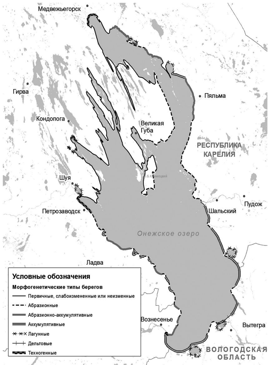
Морфогенетическая картосхема типов берегов Онежского озера (по: Исследование..., 2015)
