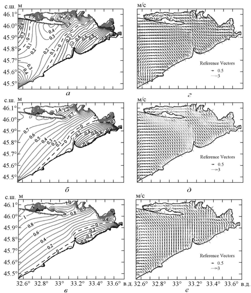
Рис. 2. Зависимость возмущений уровня моря (а–в) (м) и скоростей течений (г–е) ( \text{м}\cdot\text{с}^{-1} ) от ширины атмосферного фронта при постоянной скорости его перемещения U = 5 \text{ м}\cdot\text{с}^{-1} :
