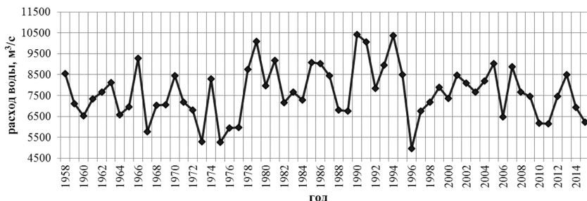
Рис. 4. Межгодовая изменчивость расходов воды
