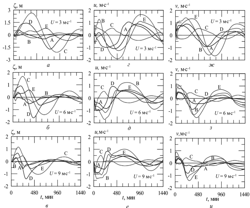
Рис. 3. Колебания уровня (а–в) и проекции u (г–е) и v (ж–и) осредненной по глубине горизонтальной скорости течения в точках А–Е (см. рис. 1) при движении фронта шириной 100 км со скоростью U = 3 \text{ м}\cdot\text{с}^{-1} (а, г, ж), U = 6 \text{ м}\cdot\text{с}^{-1} (б, д, з) и U = 9 \text{ м}\cdot\text{с}^{-1} (в, е, и)
