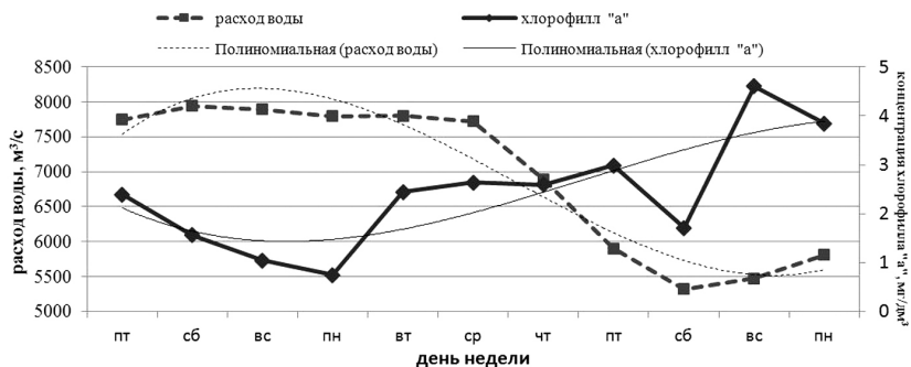
Рис. 6. Обратная связь концентрации хлорофилла (сплошная линия) и величины расходов воды (пунктирная линия) за период с 17 по 27 июля 2015 г. (эмпирические и аппроксимированные данные)
