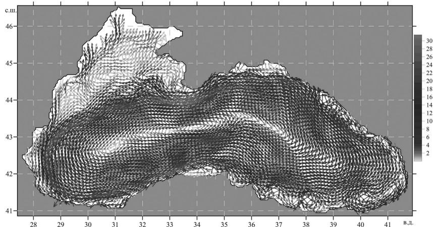
Рис. 3. Поле течений Черного моря (см/с) 10 апреля на горизонте 20 м
