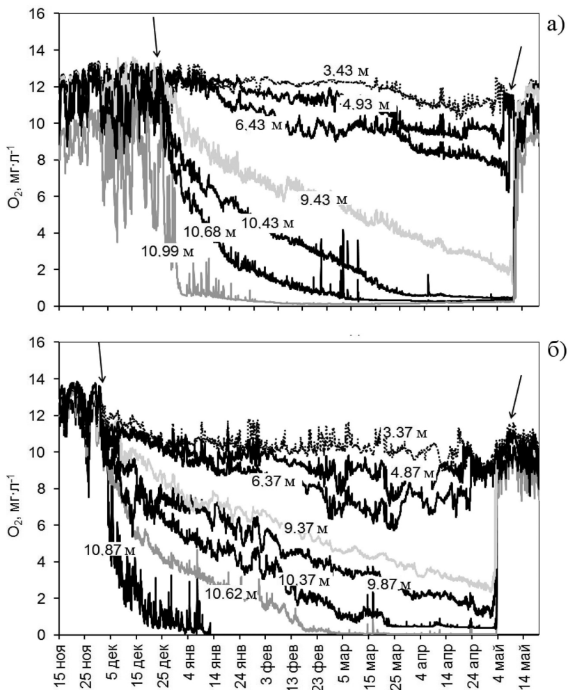
Рис. 2. Эволюция концентраций растворенного кислорода в центральной глубоководной части оз. Вендюрского:
