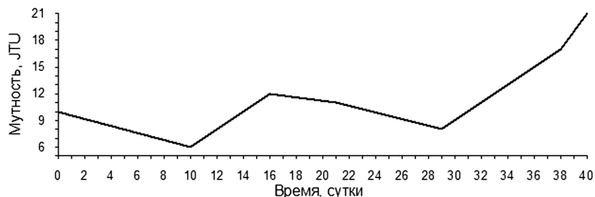
Рис. 2. Мутность воды в устье реки Томпсон [John et al., 1976]
