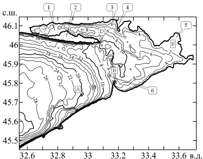
Рис. 1. Батиметрия Каркинитского залива Черного моря (в метрах):
