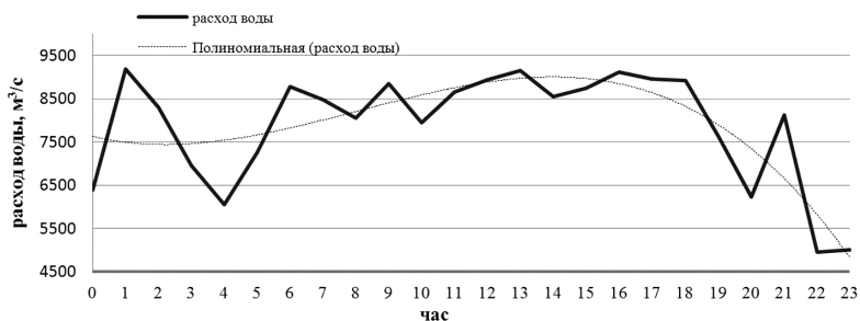
Рис. 3. Суточное регулирование расходов на ГЭС 21.07.2015 (сплошная линия – эмпирические данные, пунктирная – аппроксимация данных)
