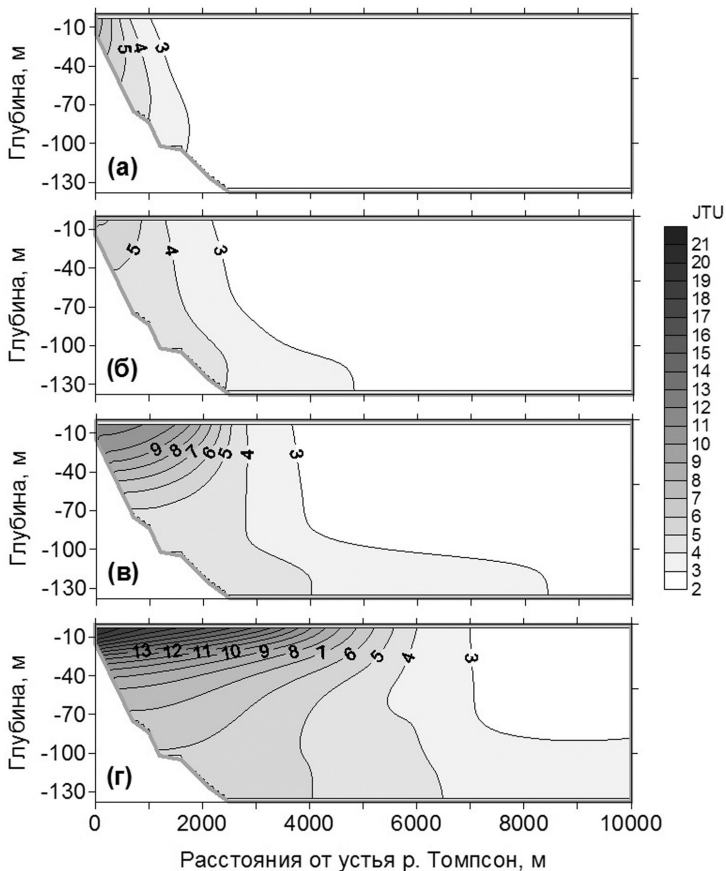
Рис. 4. Распределение мутности воды в озере Камлупс на 3 (а), 10 (б), 20 (в), 40 (г) сутки моделирования
