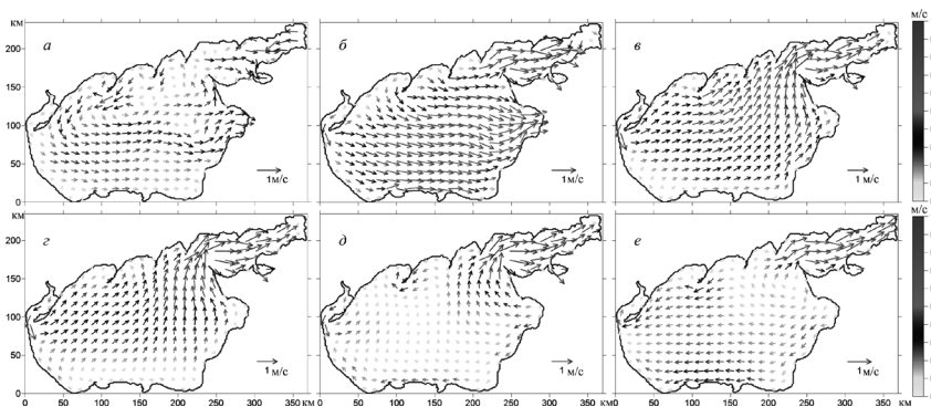
Рис. 3. Поля течений Азовского моря при установившемся движении (а), в момент прекращения действия ветра (б), через 3 ч (в), через 6 ч (г), через 9 ч (д), через 12 ч (е)
