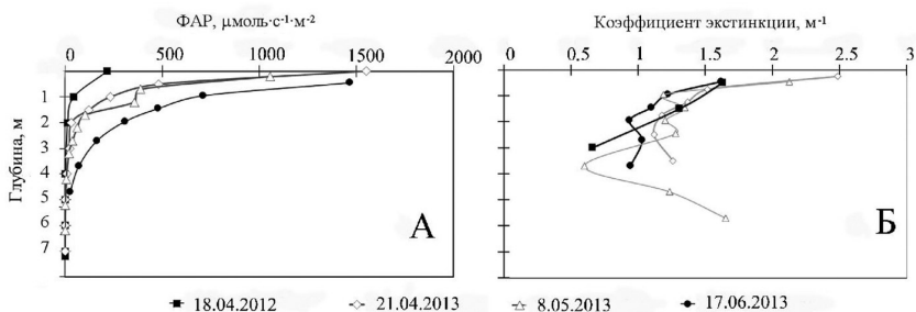
Рис. 3. Вертикальные профили распределения ФАР (А) и коэффициента экстинкции (Б) в конце периода ледостава (апрель) и на этапе раннего лета (май, июнь)
