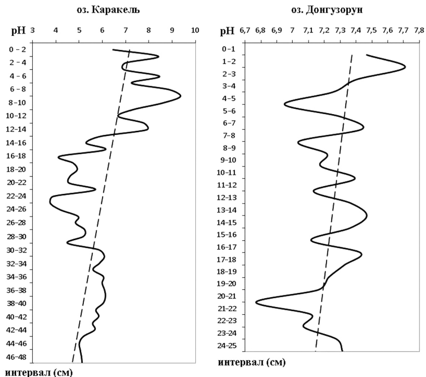
Рис. 2. Долговременные изменения численных значений рН в двух озерах Центрального Кавказа
