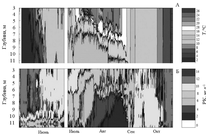
Рис. 2. Формирование «запирающей» стратификации (А) и придонной бескислородной зоны (Б) в оз. Вендюрском летом 2010 г.
