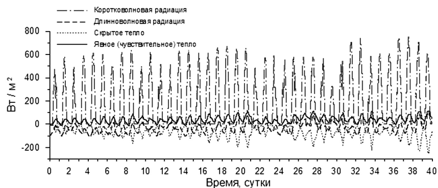
Рис. 3. Компоненты тепловых потоков, рассчитанные на основе атмосферных данных метеорологической станции г. Камлупс в период с 01.04.2015 по 10.05.2015 г. (местное стандартное время)
