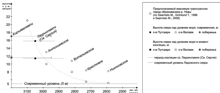
Рис. 2. График обособления малых озер островов Валаам, Путсаари и северо-западного побережья Ладожского озера от Ладоги
