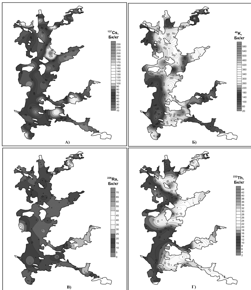
Распределение удельной активности радионуклидов в донных отложениях оз. Каменного, Бк/кг:
