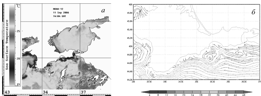
Рис. 3. Поле температуры поверхности моря ( ^{\circ}\text{C} ) по данным спутника NOAA ( а ) и карта течений (см/с) на верхнем расчетном горизонте ( б ) на 11.09.06
