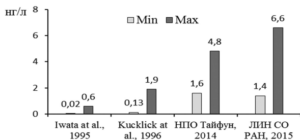
Рис. 3. Диапазоны суммарных концентраций обнаруженных конгенов ПХБ в поверхностной воде оз. Байкал в 1995–1996 и 2014–2015 гг.
