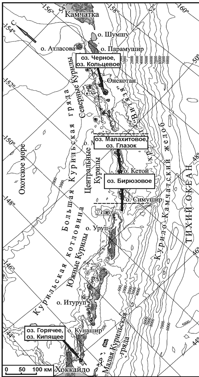
Расположение кратерных озер Курильских островов
