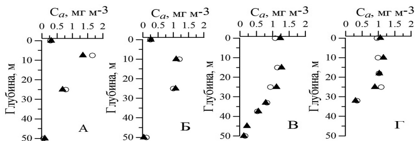
Рис. 2. Вертикальное распределение концентрации хлорофилла а в слое 0–50 м в сентябре (А, Б) и декабре (В, Г) 2015 г.:
