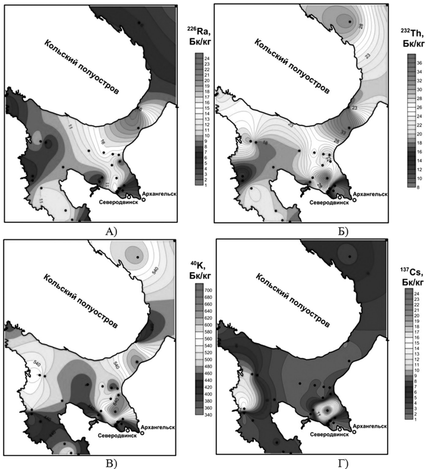
Распределение активности изотопов ^{226}\text{Ra} , ^{232}\text{Th} , ^{40}\text{K} , ^{137}\text{Cs} (Бк/кг) в донных осадках Белого моря
