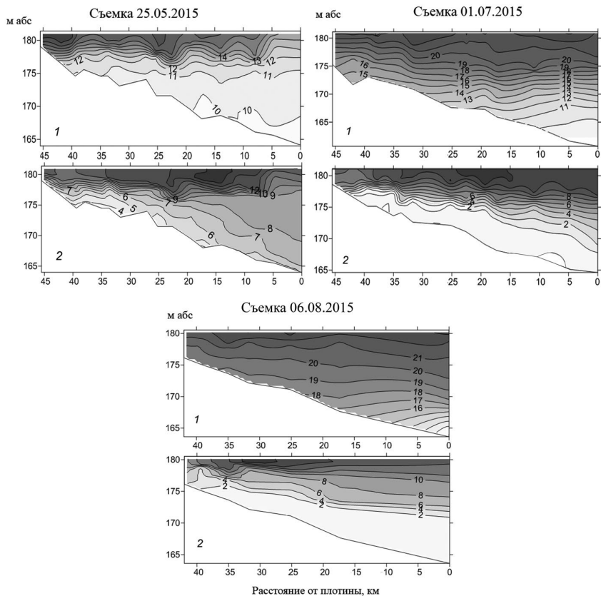
Рис. 2. Распределение температуры воды (°C) и растворенного кислорода (мг/л) по данным гидролого-гидрохимических съемок
