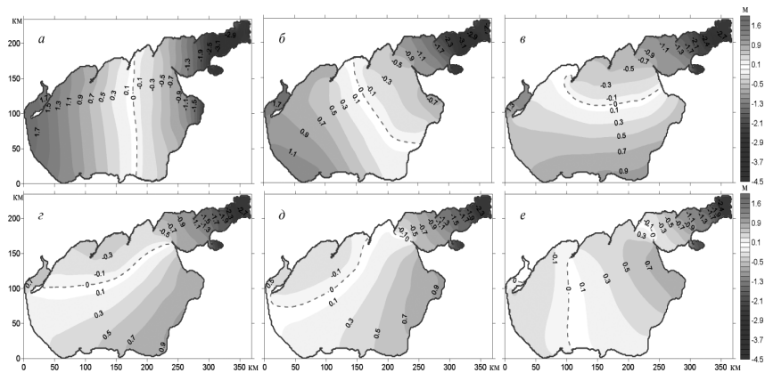
Рис. 1. Изолинии уровня (м) Азовского моря при установившемся движении (а), в момент прекращения действия ветра (б), через 3 ч (в), через 6 ч (г), через 9 ч (д), через 12 ч (е)
