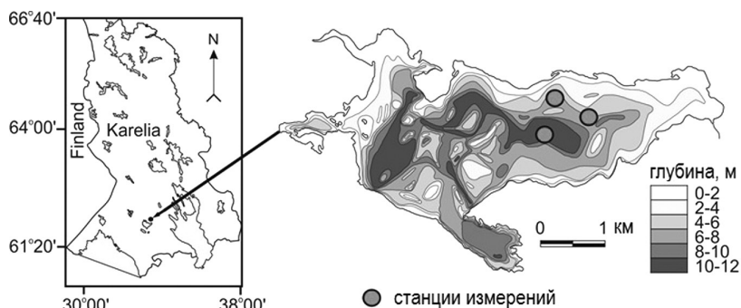
Рис. 1. Батиметрия оз. Вендюрского и расположение станций измерений
