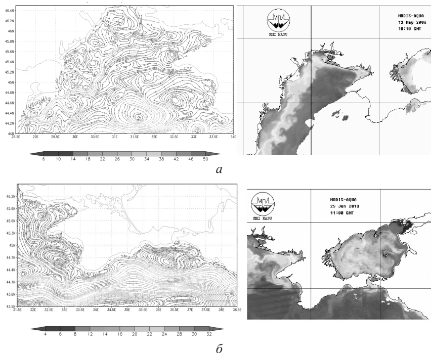
Рис. 2. Карты течений (см/с) на верхнем расчетном горизонте и снимки полей концентрации хлорофилла по данным MODIS: а – 13.05.06; б – 25.06.13
