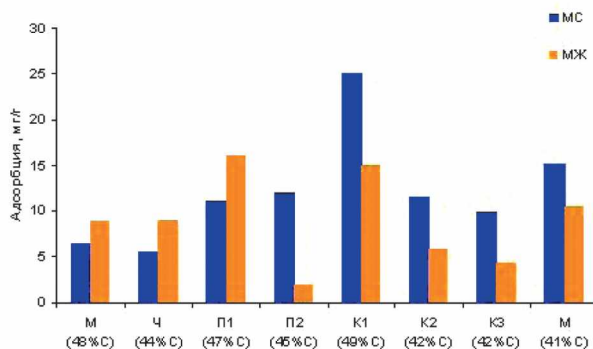
Рис. 27. Сорбционная активность шунгитовых пород по отношению к анионным (МК) и катионным (МС) красителям
