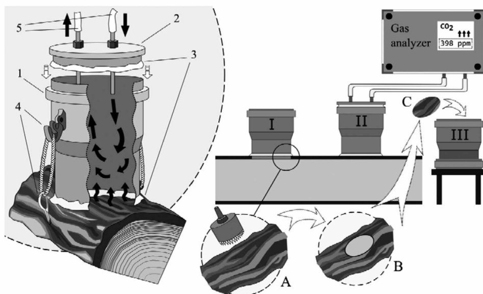
Рис. 38. Схема метода: I – измерение общего потока \text{CO}_2 с ненарушенной поверхностью валежа (A); II – измерение потока \text{CO}_2 с оголенной древесины (B); III – измерение потока \text{CO}_2 со срезанной коры (C). (1) камера, (2) крышка камеры, (3) герметик, (4) специальный крепеж, (5) трубки, соединенные с газоанализатором \text{CO}_2
